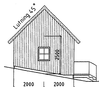
Fasad mot väster (mot vägen)
