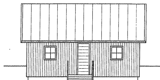
Fasad mot söder
