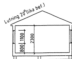
Sektion genom tillbyggnad
