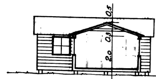
SEKTION
